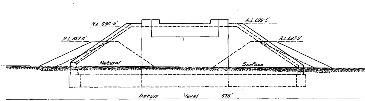
- ELEVATION -
